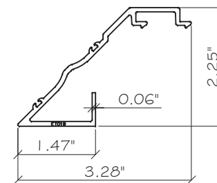
E13 EXTERIOR CORNER FIN GW 7000-750 ALUM. 6063-T6
