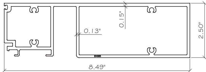
E10 SILL HORIZONTAL FRONT ALP-026 ALUM. 6063-T6
