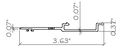
E12 FIN GW-7000-498 ALUM. 6063-T6
