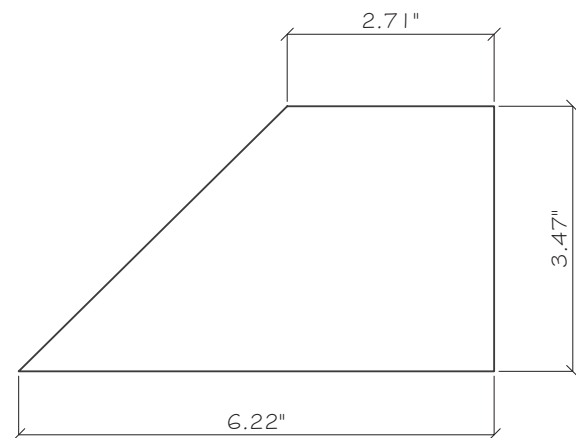
E46 3/8" THK. ALUM. PLATE ALUM. 6061-T6
