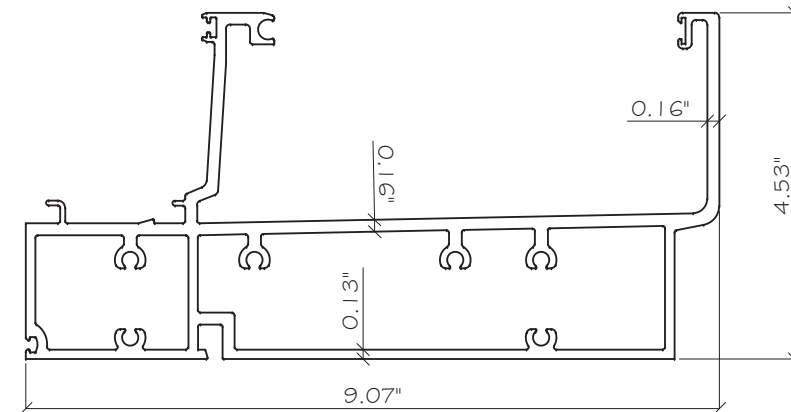
E9 GUTTER FRONT ALP-021 ALUM. 6063-T6
