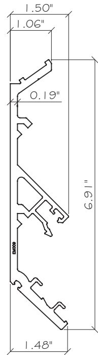
E3 FEMALE MULLION GW-7000-167 ALUM. 6063-T6
