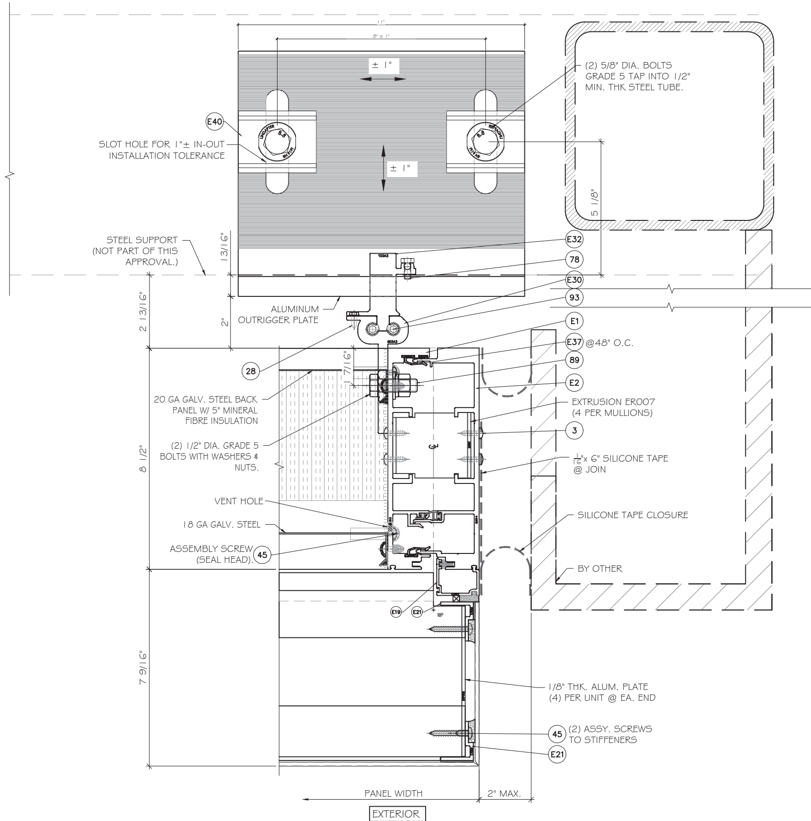
1 PLAN DETAIL. D28 SCALE: 1'-0"=1'-0"
