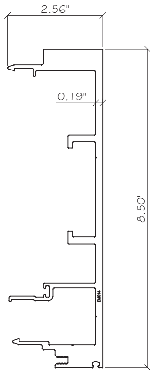
E2 MALE MULLION GW-7000-191 ALUM. 6063-T6
