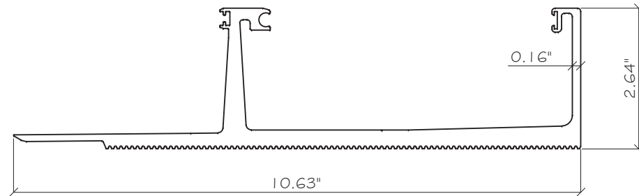
E8 SUBSILL ALP-036 ALUM. 6061-T6
