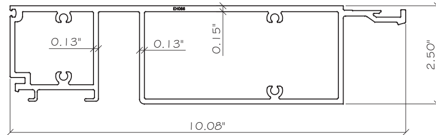
E11 SILL HORIZONTAL FRONT ALP-031 ALUM. 6063-T6
